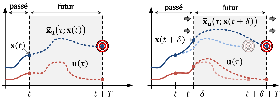
FIGURE 1.3 – Principe de base de la commande prédictive.
