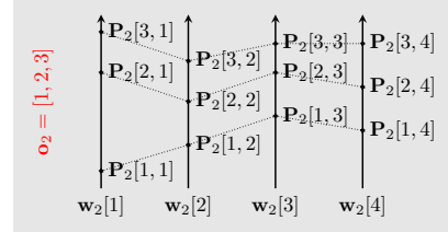
(b) swap_orders
