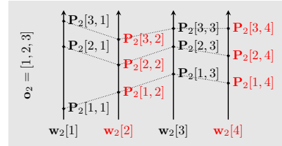
(d) mix_criteria_and_weights
