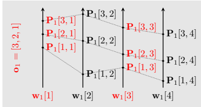
(d) mix_criteria_and_weights
