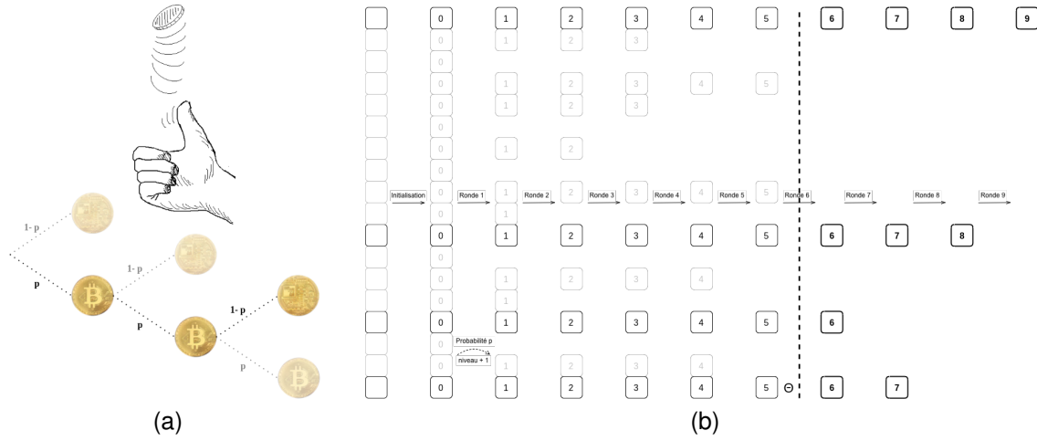
FIGURE 1: Illustration des deux étapes de notre algorithme FTK_{CE} .
